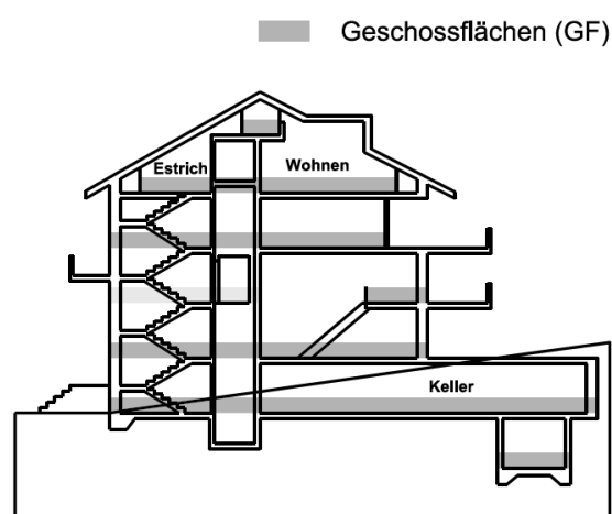
Schnitt:
