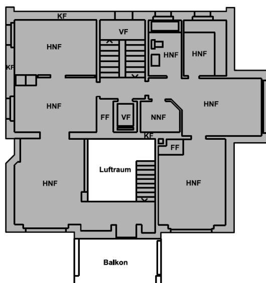
Grundriss 1. Obergeschoss:
