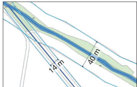
Bsp. Gewässerraumplan NRP Ingenieure
